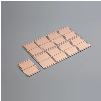
Silicon nitride AMB substrate with patterned copper
